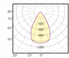
SYMMETRISCHE LINSE UGR<19 SYMMETRIC LENS UGR<19
